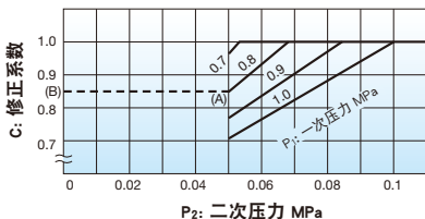
Cv 修正值
